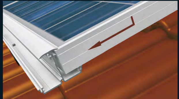
Solarmodul in das untere Horizontalprofil gleiten lassen
